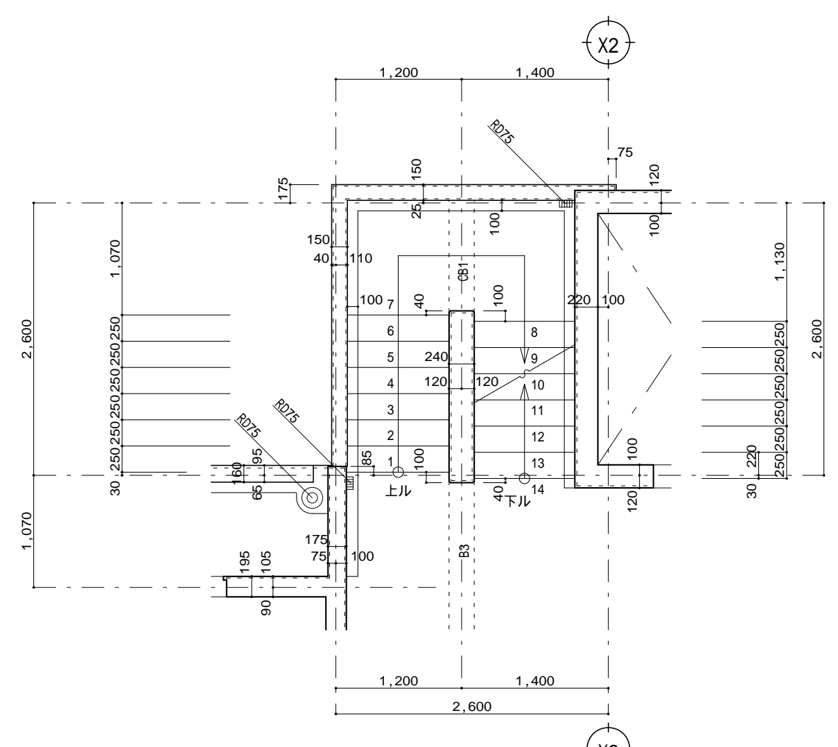
A階段 2~5階平面図 S=1:50
