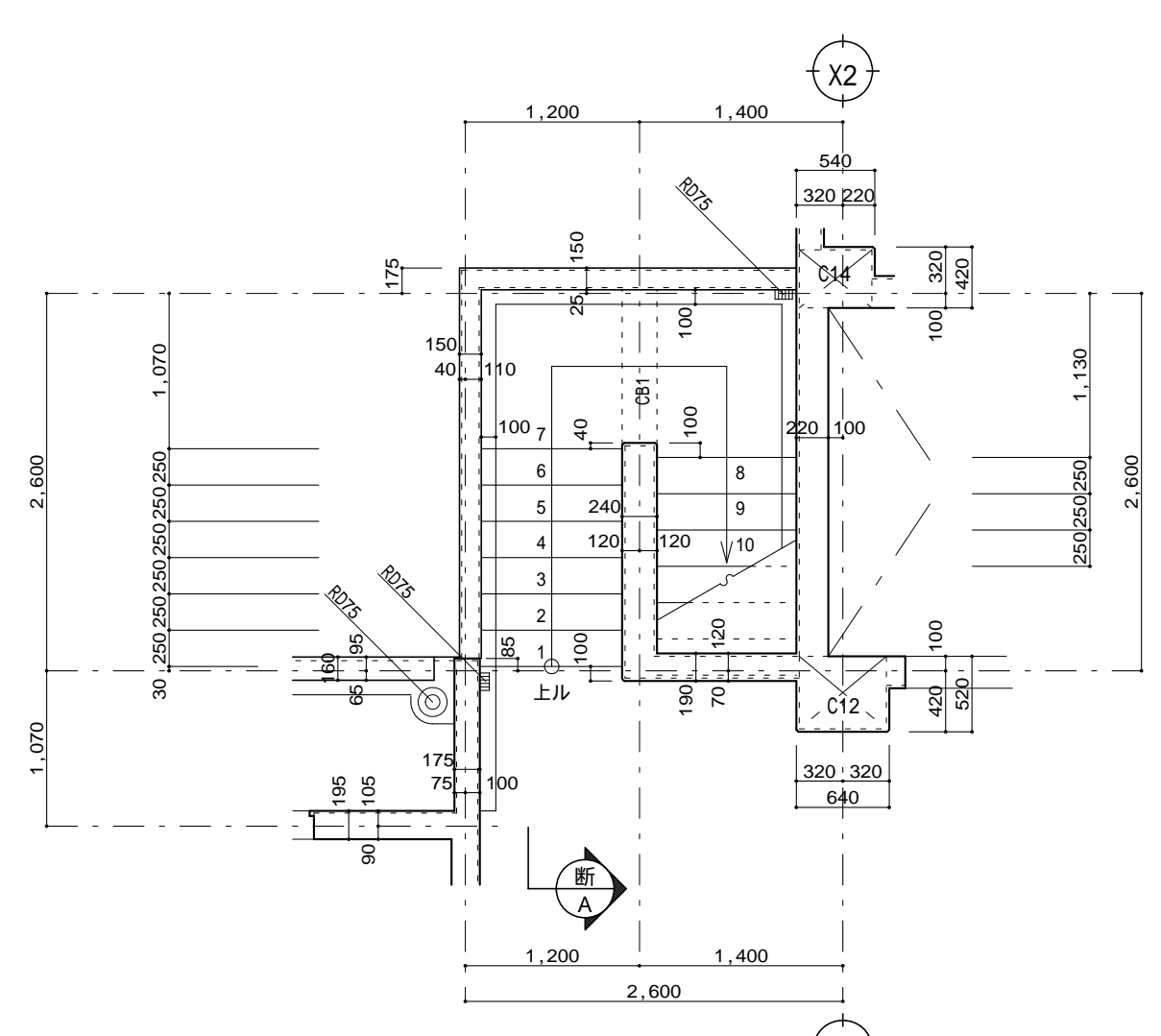
A階段 1階平面図 S=1:50
