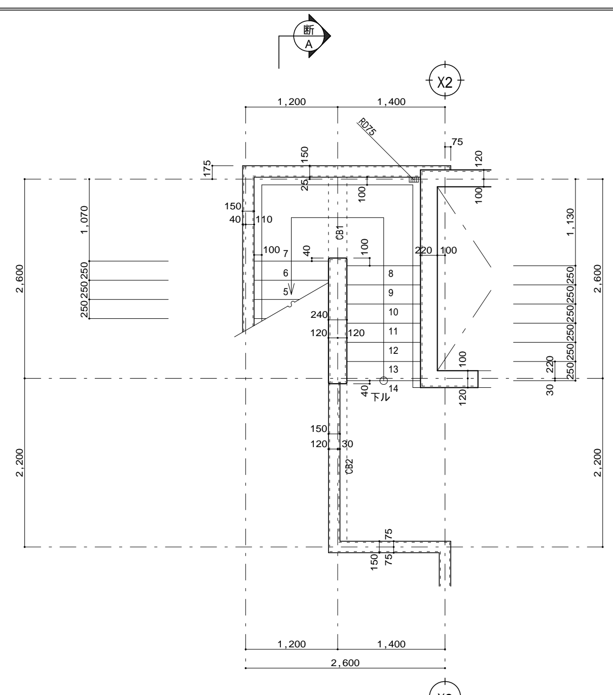
A階段 6階平面図 S=1:50
